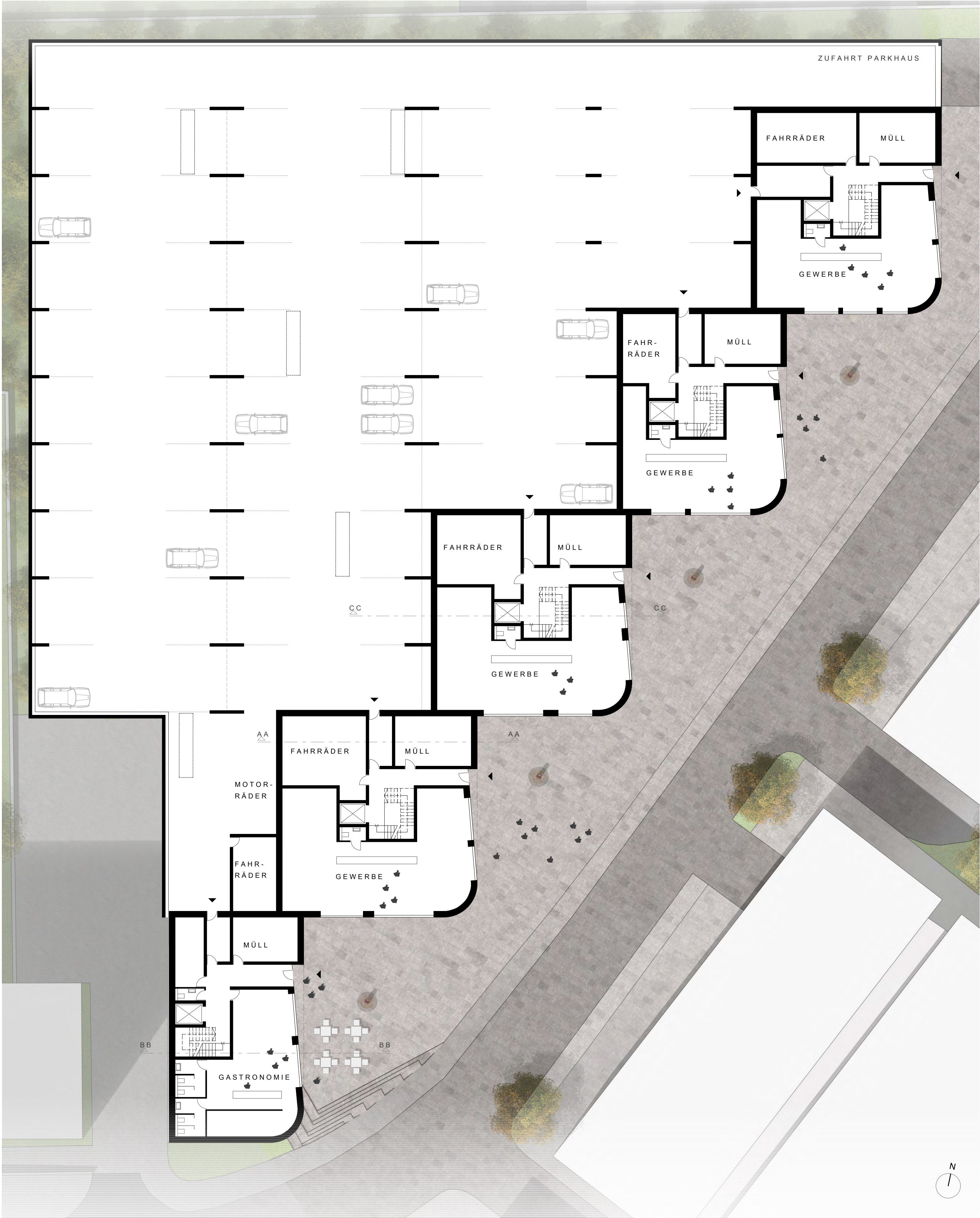
GRUNDRISS ERDGESCHOSS M 1.200
